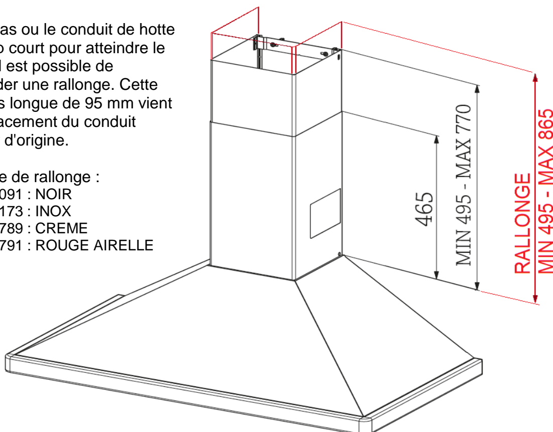
CONDUIT INFERIEUR
